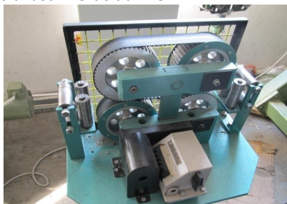
Uređaj za premotavanje kablova i trakasti merač dužine
